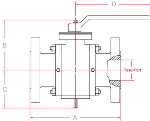
Serie 82 (Clase 150) • Series 82 (Class 150)
