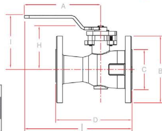
Dimensiones • Dimensions
