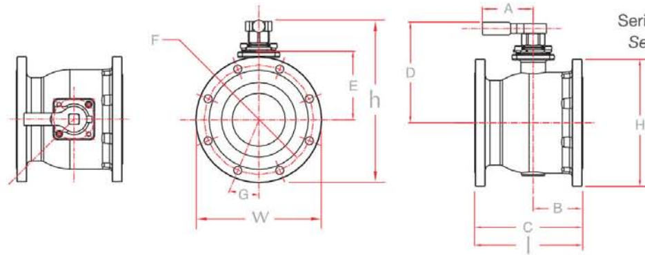
Serie 150 • Series 150
