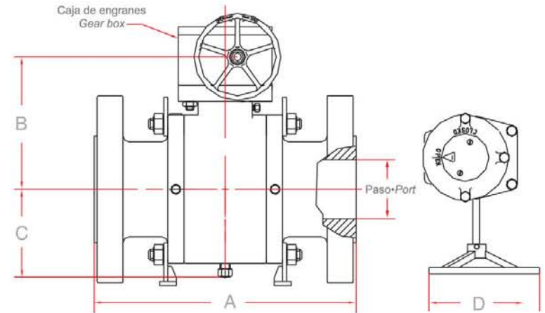
Serie 83 (Clase 300) • Series 83 (Class 300)
