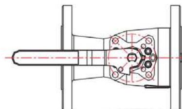
Dimensiones • Dimensions
