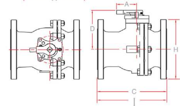
Serie 302 • Series 302
