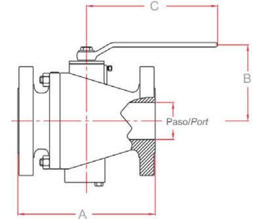
Dimensiones • Dimensions
